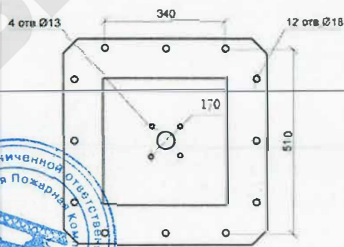
Присоединительные размеры фланца генератора пены
