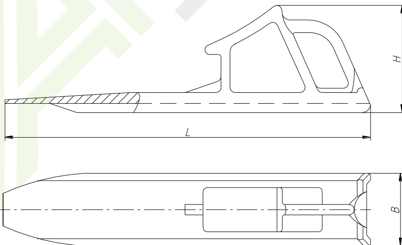
Рисунок 1– Башмак БК-1А
