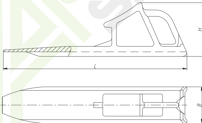
Рисунок 1 – Башмак БК-1Л
