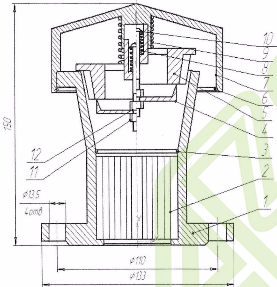
Рисунок 1: СМДК-50АА – устройство.
