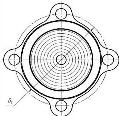
1 – огнепреграждающий элемент; 2 – корпус Рисунок 1 – Огнепреградители ОП-DN
